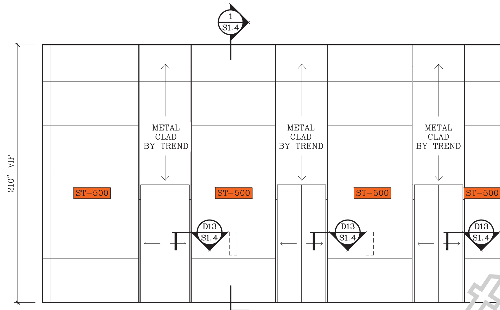
S ELEVATION SCALE: 1/4"=1'-0"
