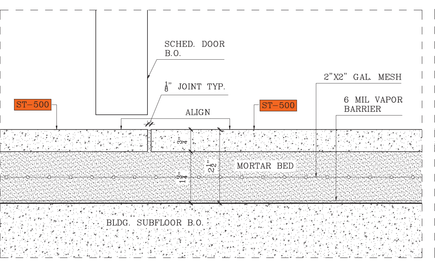
D9 VERTICAL DETAIL SCALE: 6"=1'-0"
