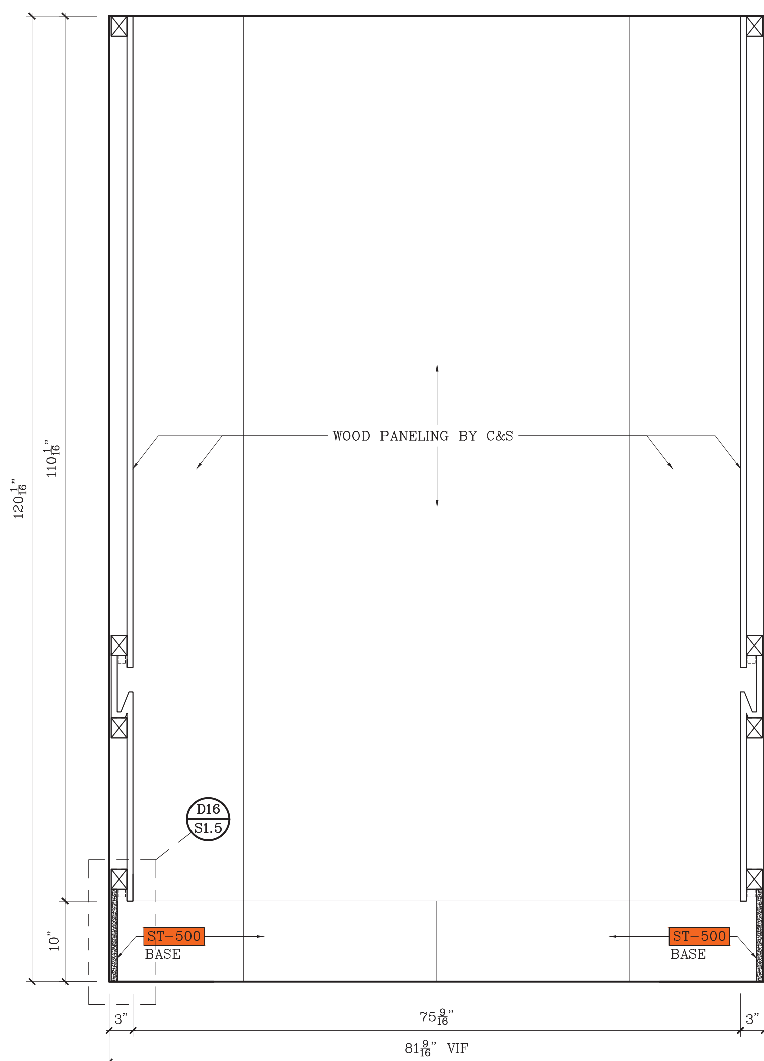
A ELEVATION SCALE: 1"=1'-0"
