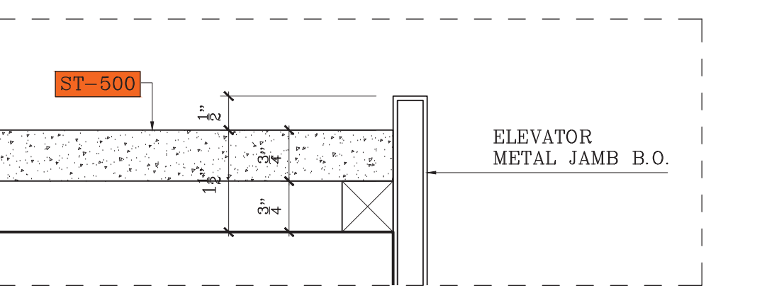
D13 PLAN DETAIL SCALE: 6"=1'-0"
