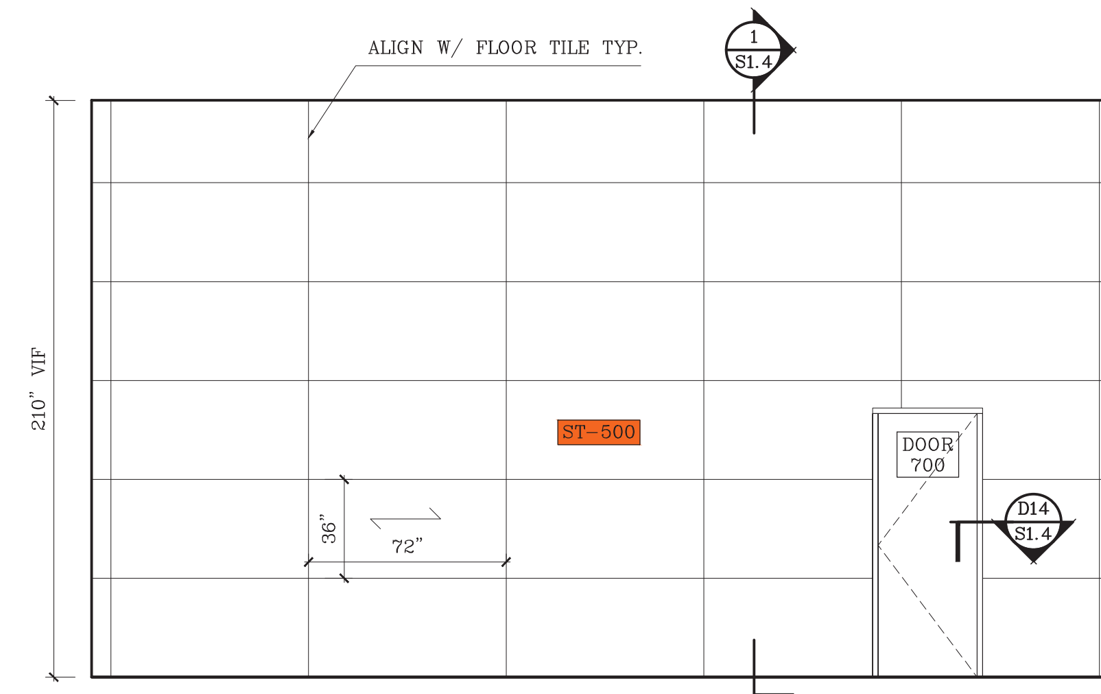
T ELEVATION SCALE: 1/4"=1'-0"
