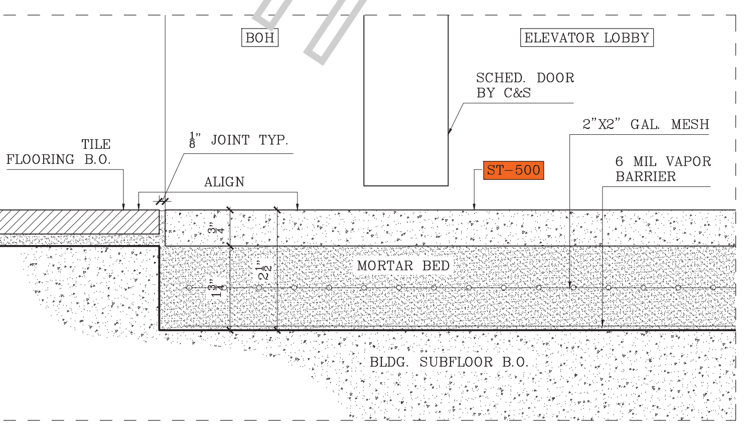
D10 VERTICAL DETAIL SCALE: 6"=1'-0"
