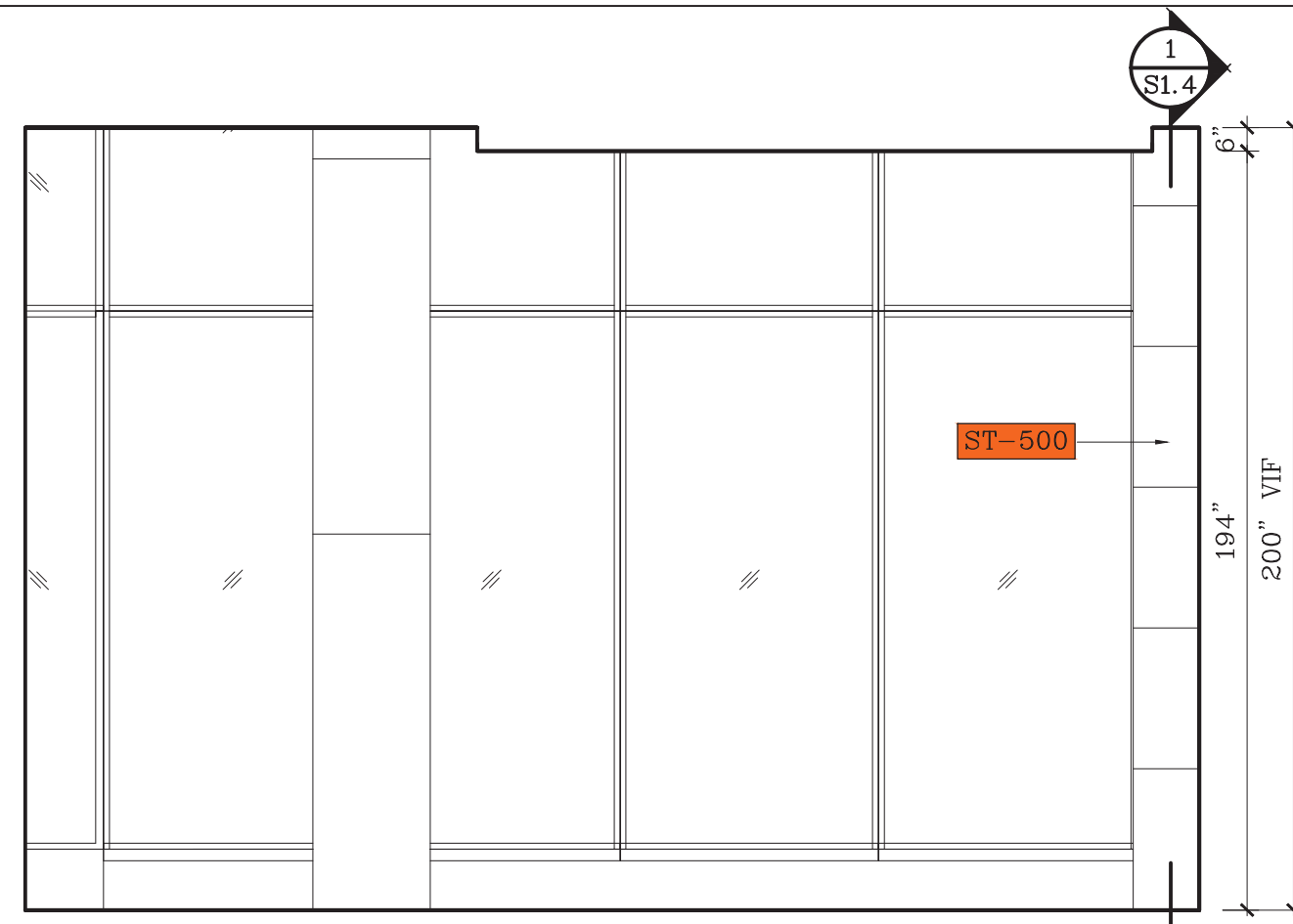
F ELEVATION SCALE: 1/4"=1'-0"
