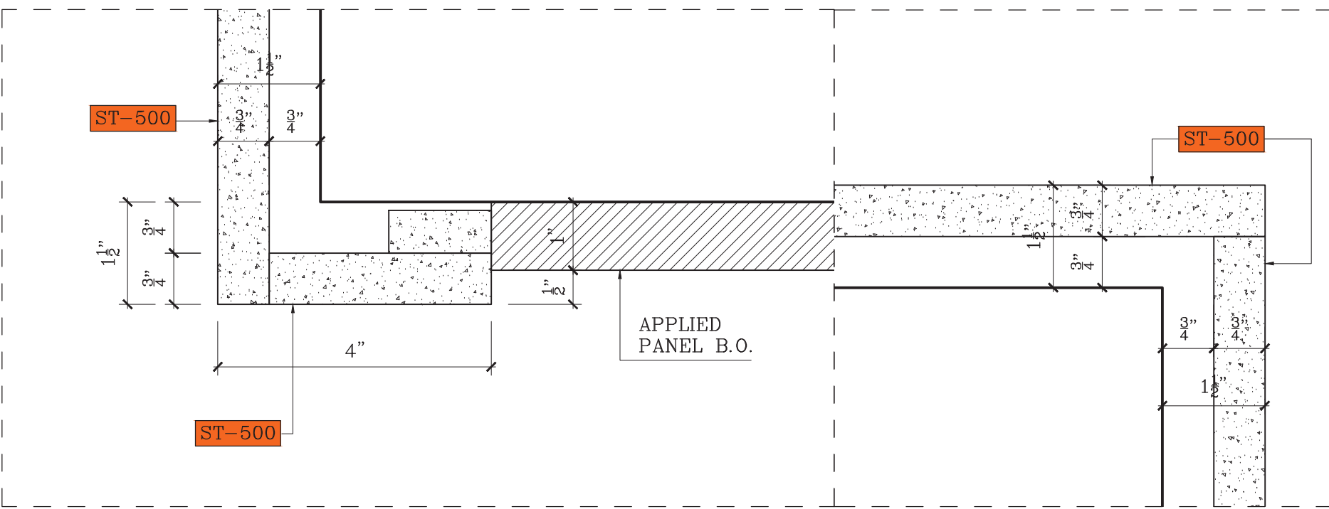
D1 PLAN DETAIL SCALE: 6"=1'-0"
