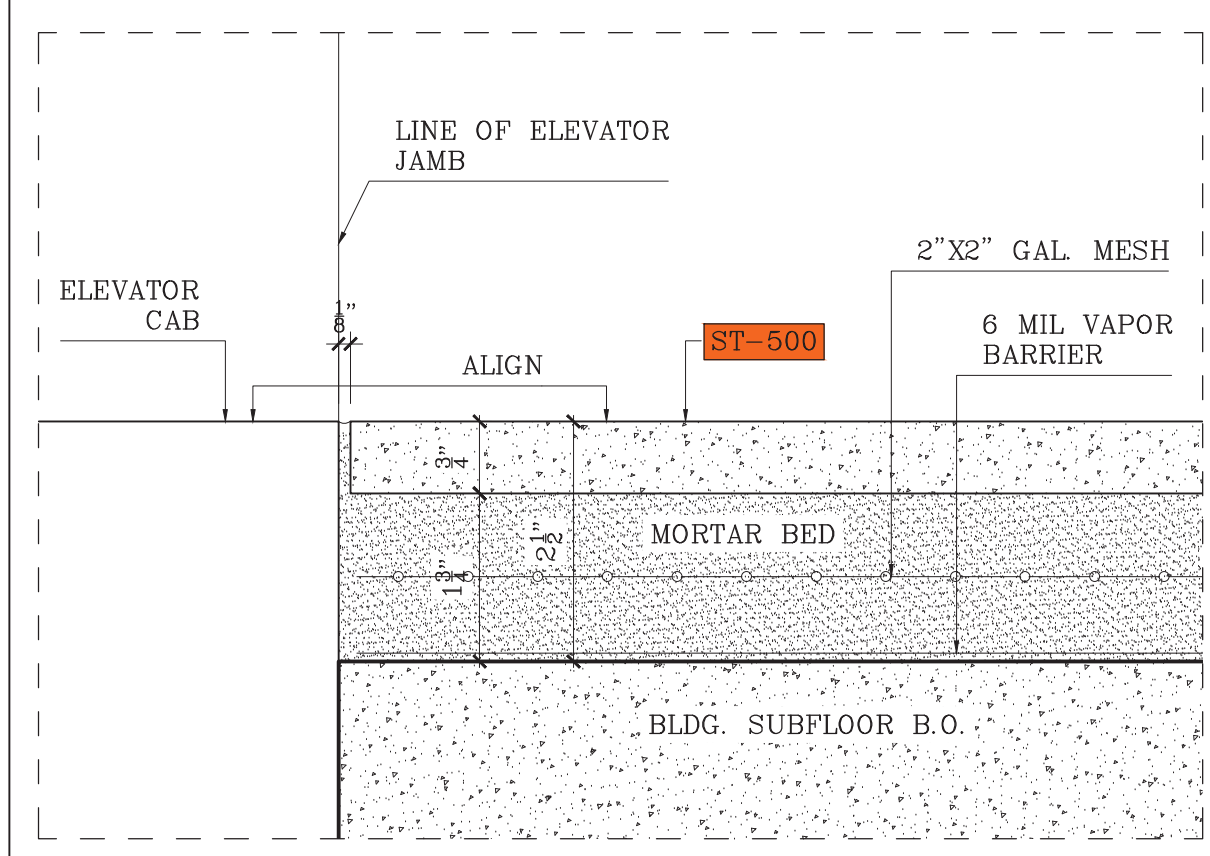
D7 VERTICAL DETAIL SCALE: 6"=1'-0"
