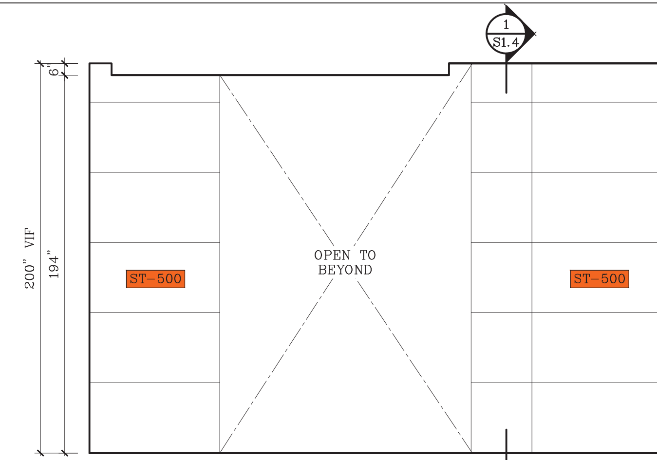
H ELEVATION SCALE: 1/4"=1'-0"
