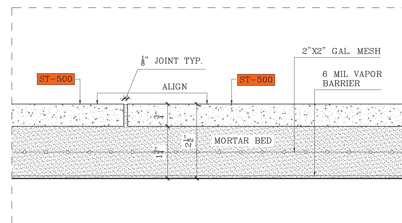
D15 VERTICAL DETAIL SCALE: 6"=1'-0"
