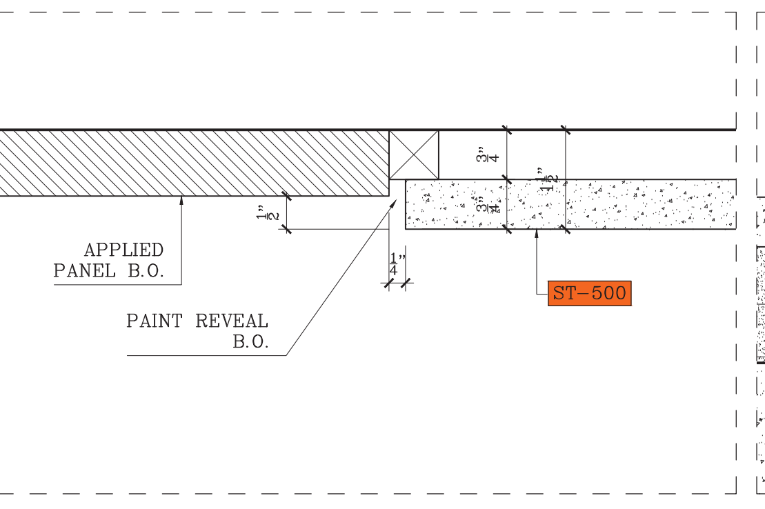
D5 PLAN DETAIL SCALE: 6"=1'-0"
