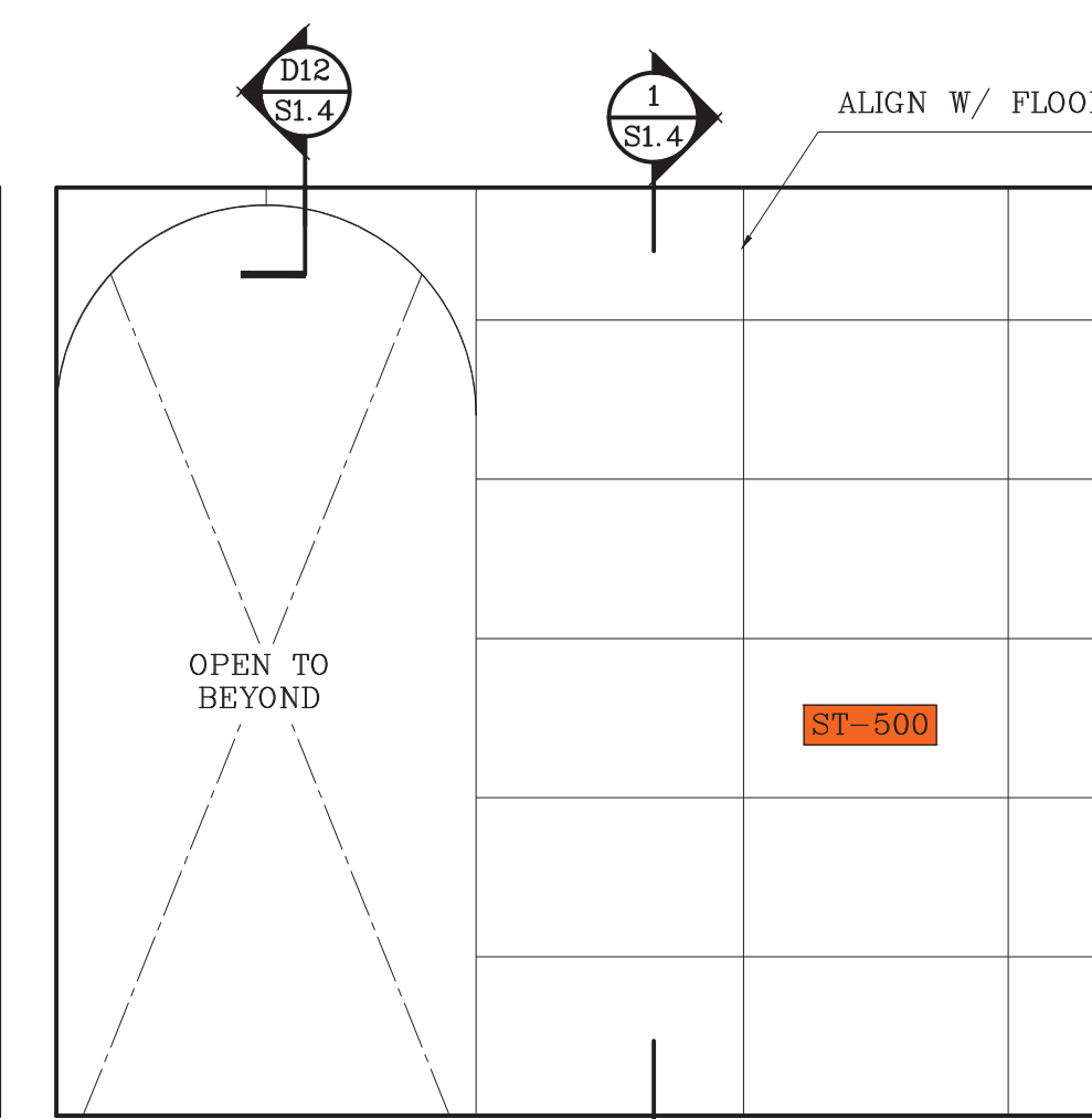
Q ELEVATION SCALE: 1/4"=1'-0"
