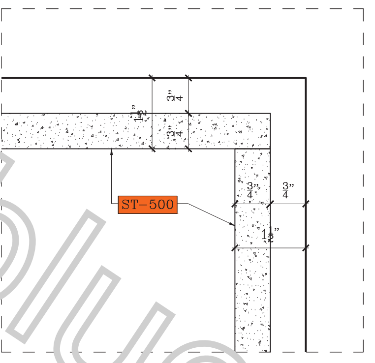
D4 PLAN DETAIL SCALE: 6"=1'-0"
