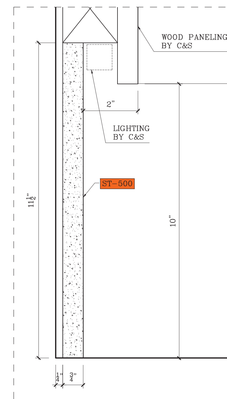
D16 VERTICAL DETAIL SCALE: 6"=1'-0"
