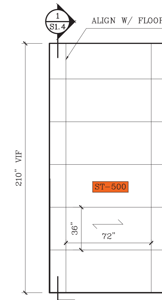
U ELEVATION SCALE: 1/4"=1'-0"
