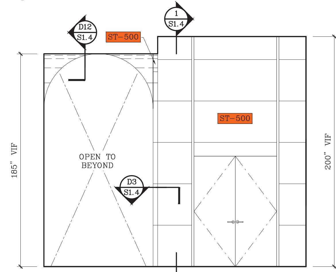
J ELEVATION SCALE: 1/4"=1'-0"
