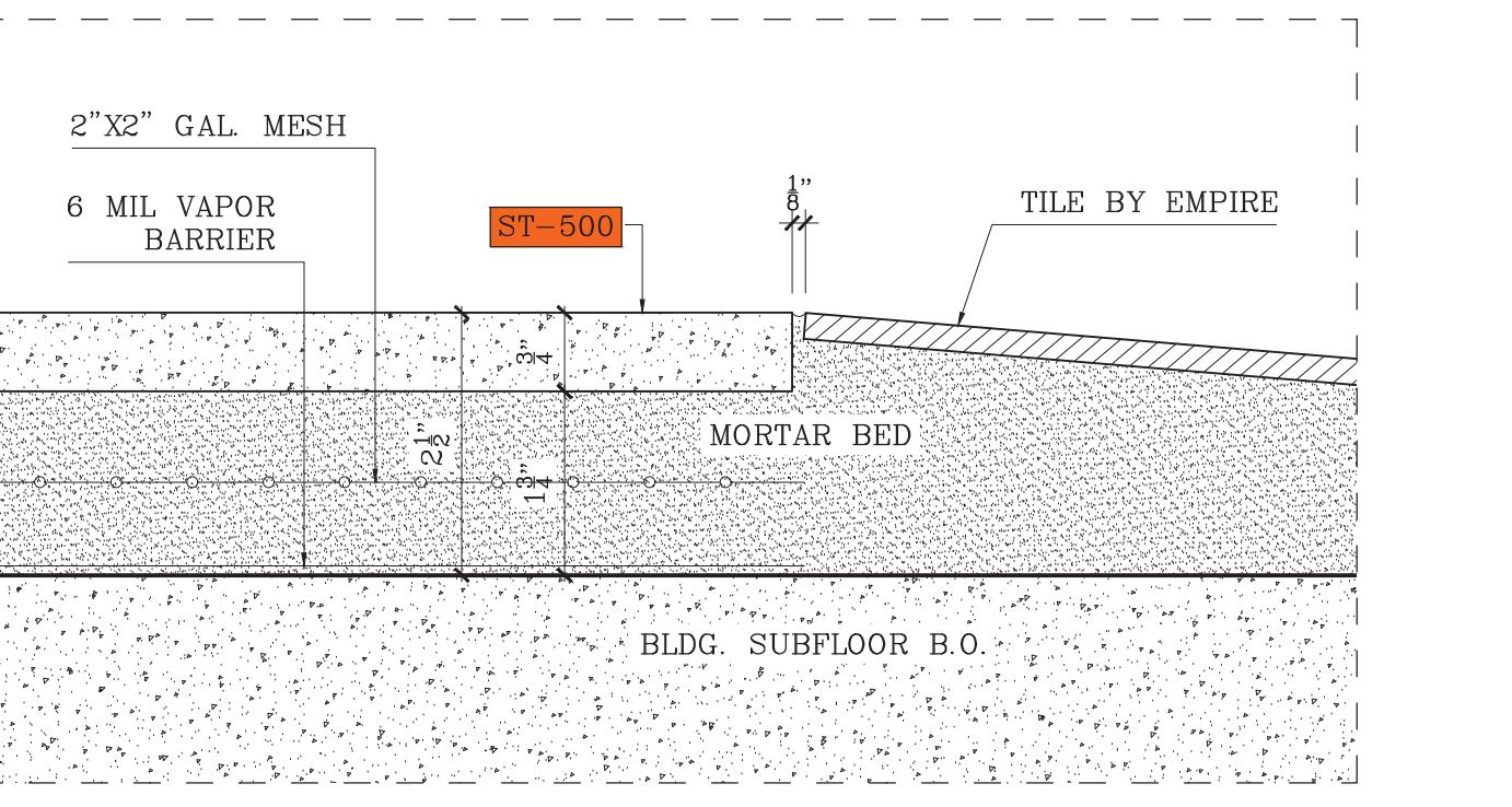
D6 VERTICAL DETAIL SCALE: 6"=1'-0"
