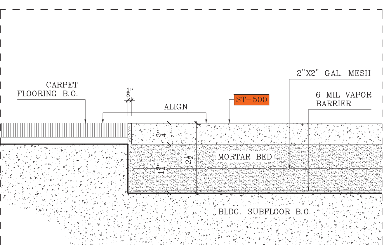
D8 VERTICAL DETAIL SCALE: 6"=1'-0"
