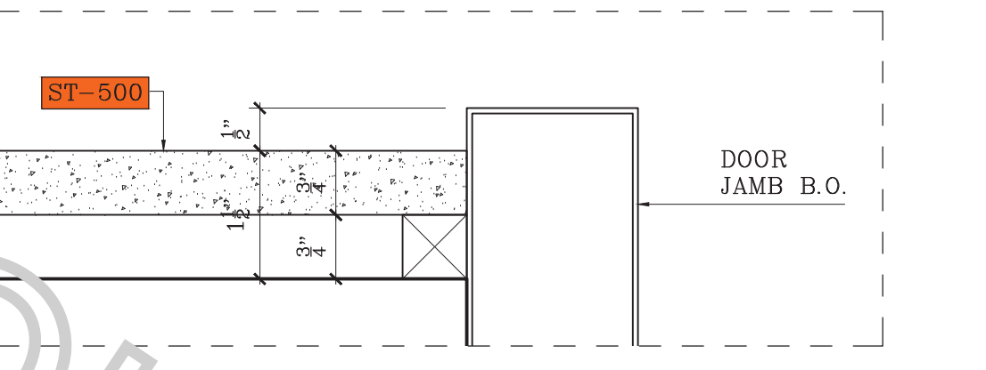
D14 PLAN DETAIL SCALE: 6"=1'-0"
