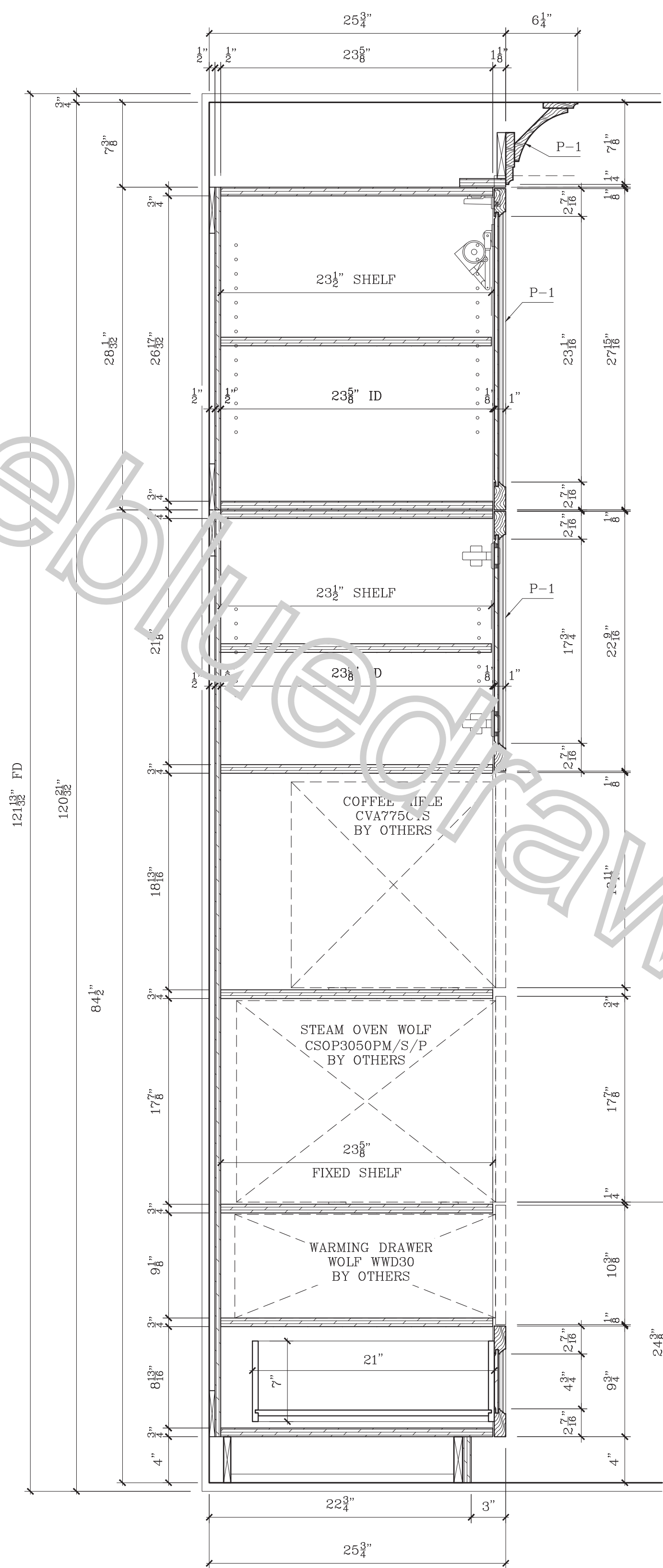
12 VERTICAL SECTION SCALE: 1-1/2"=1'-0"
