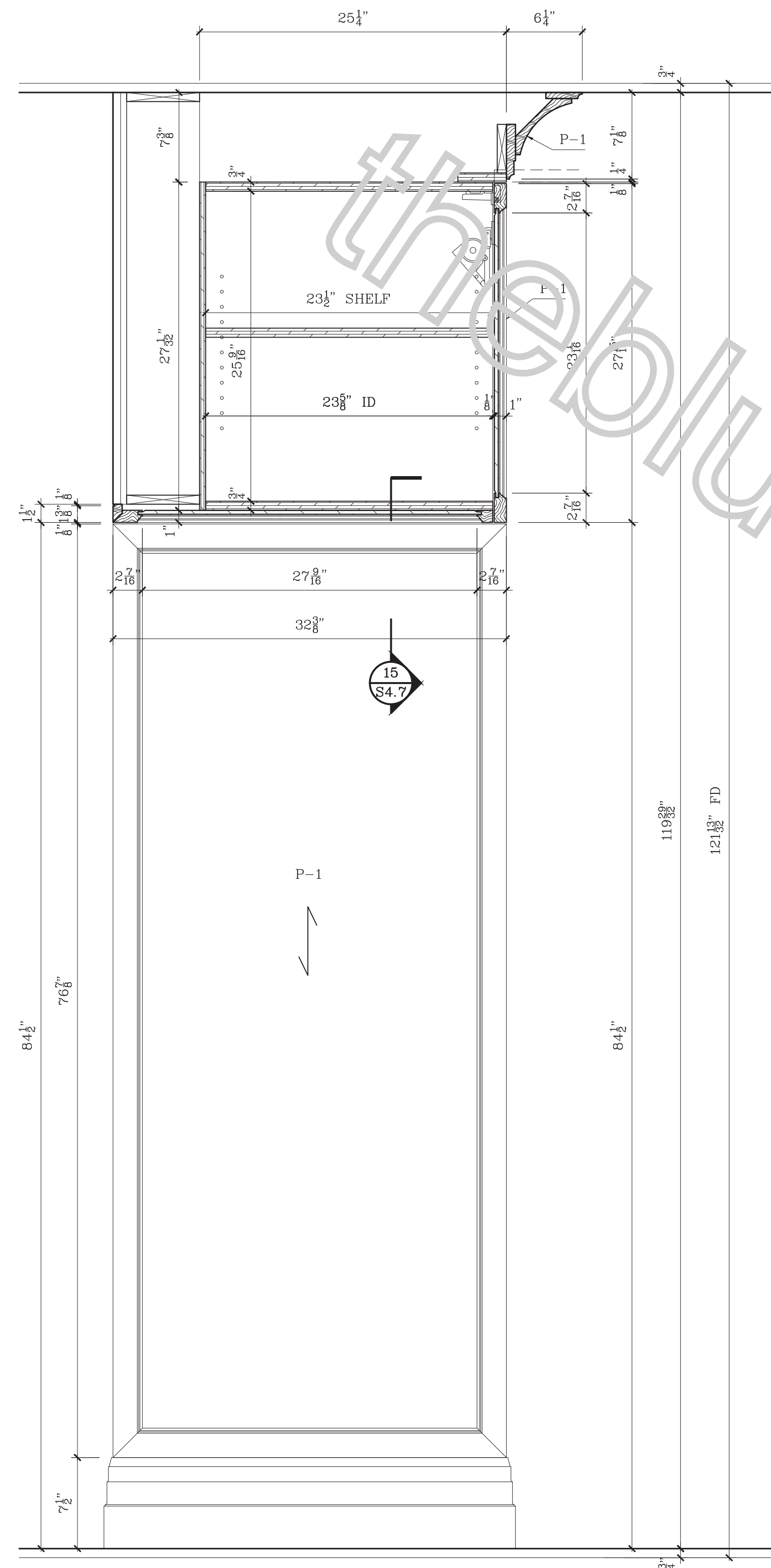
14 VERTICAL SECTION SCALE: 1-1/2"=1'-0"
