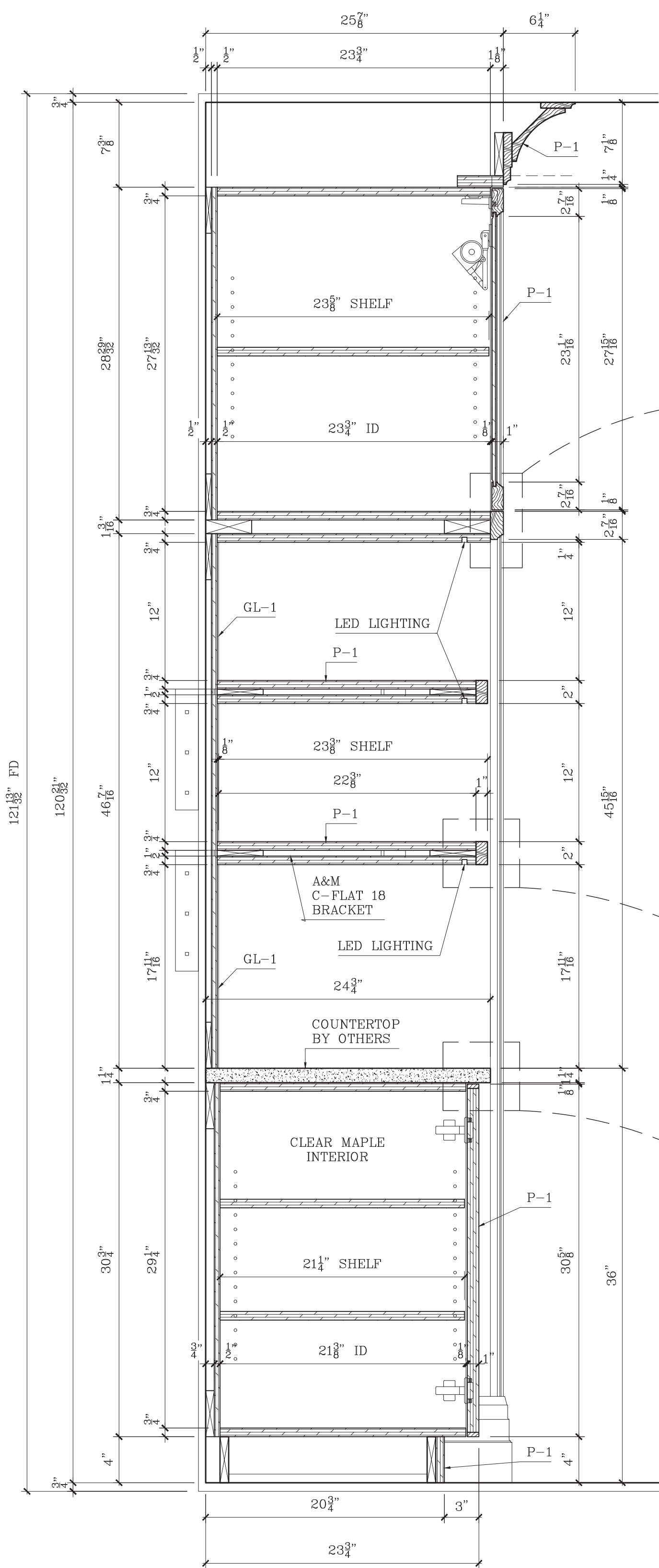
7 VERTICAL SECTION SCALE: 1-1/2"=1'-0"
