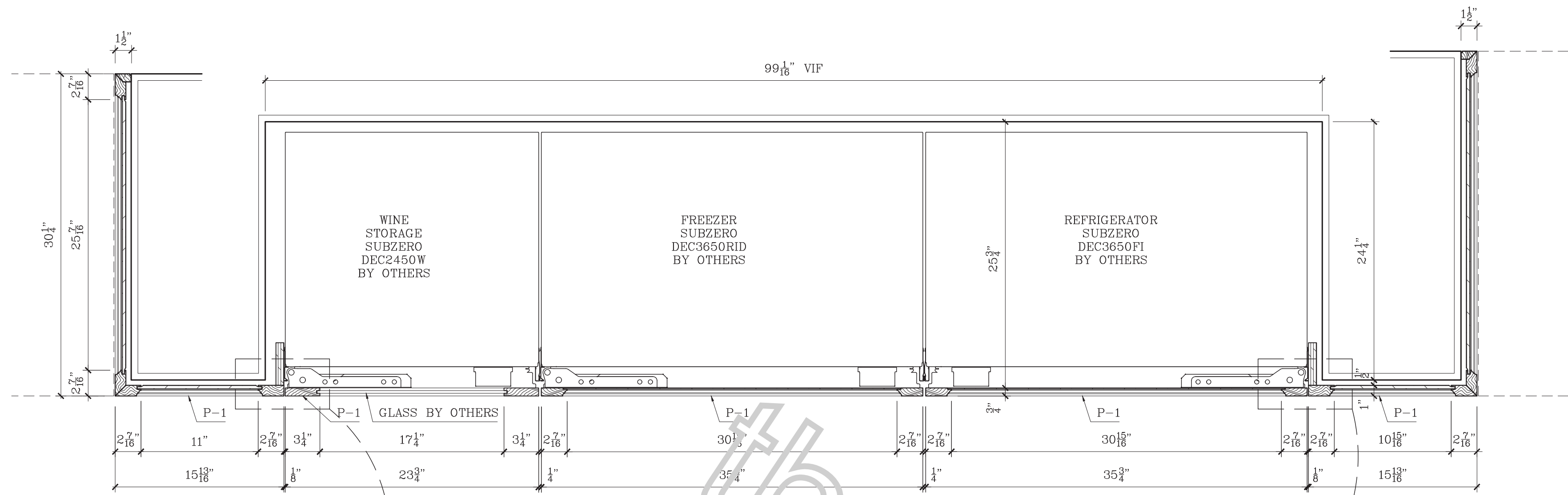
3 PLAN SECTION SCALE: 1-1/2"=1'-0"
