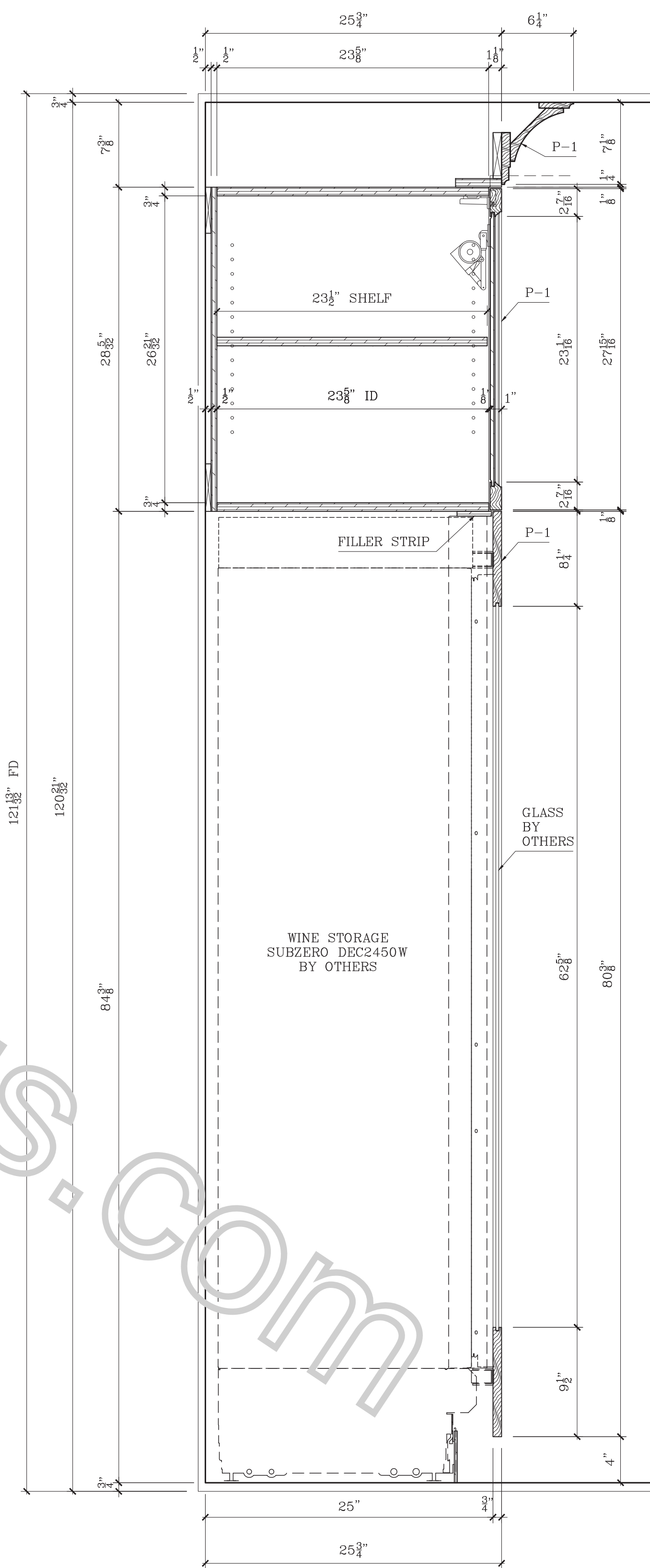
13 VERTICAL SECTION SCALE: 1-1/2"=1'-0"
