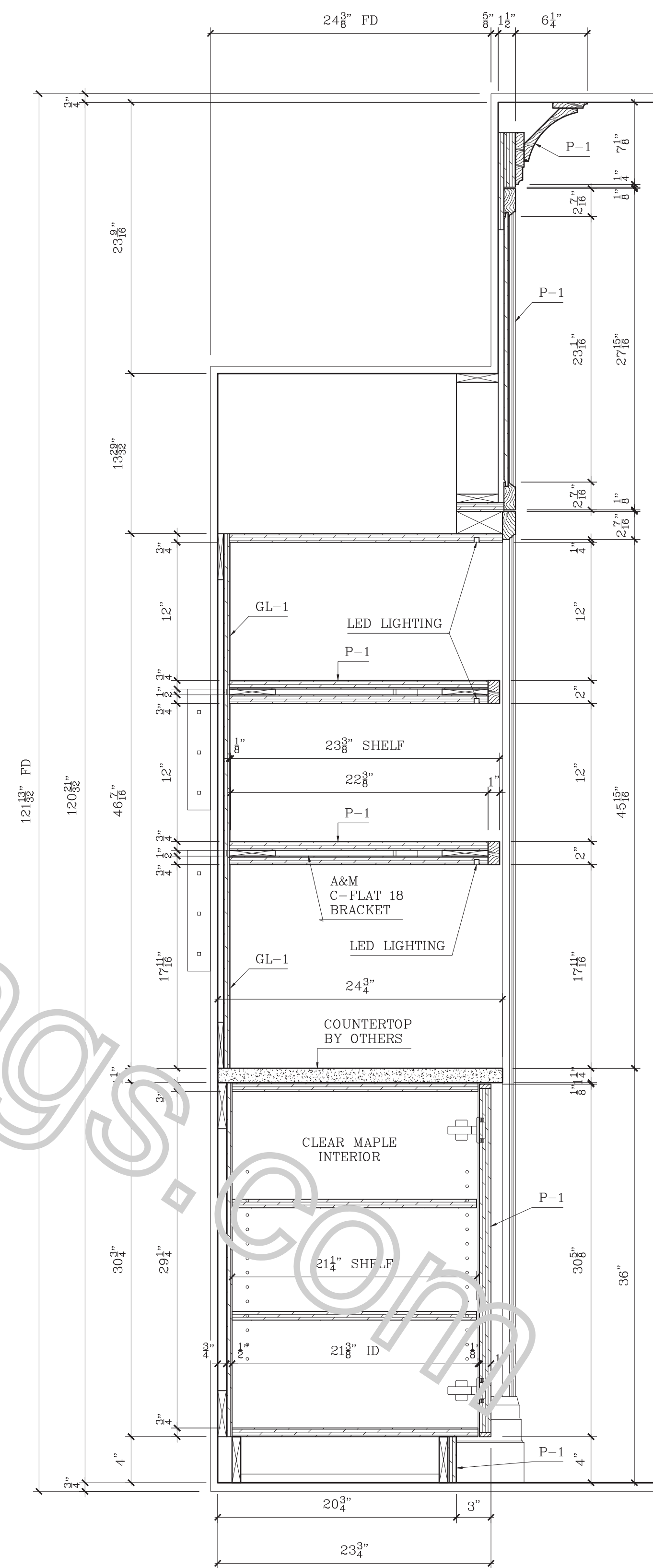
8 VERTICAL SECTION SCALE: 1-1/2"=1'-0"
