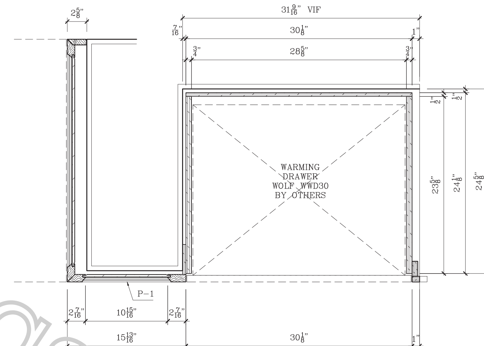
5 PLAN SECTION SCALE: 1-1/2"=1'-0"
