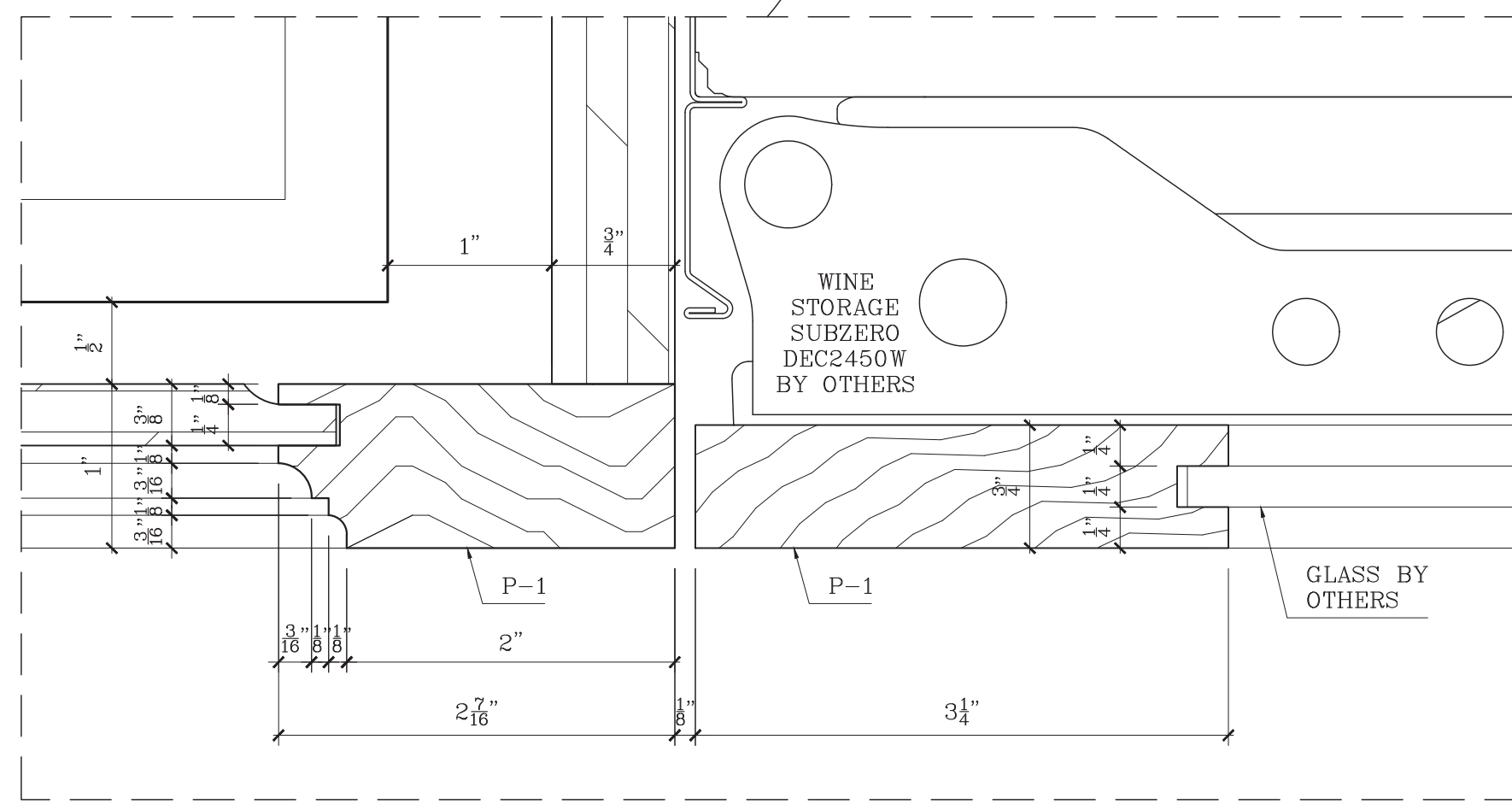
3 PLAN SECTION SCALE: 1-1/2"=1'-0"
