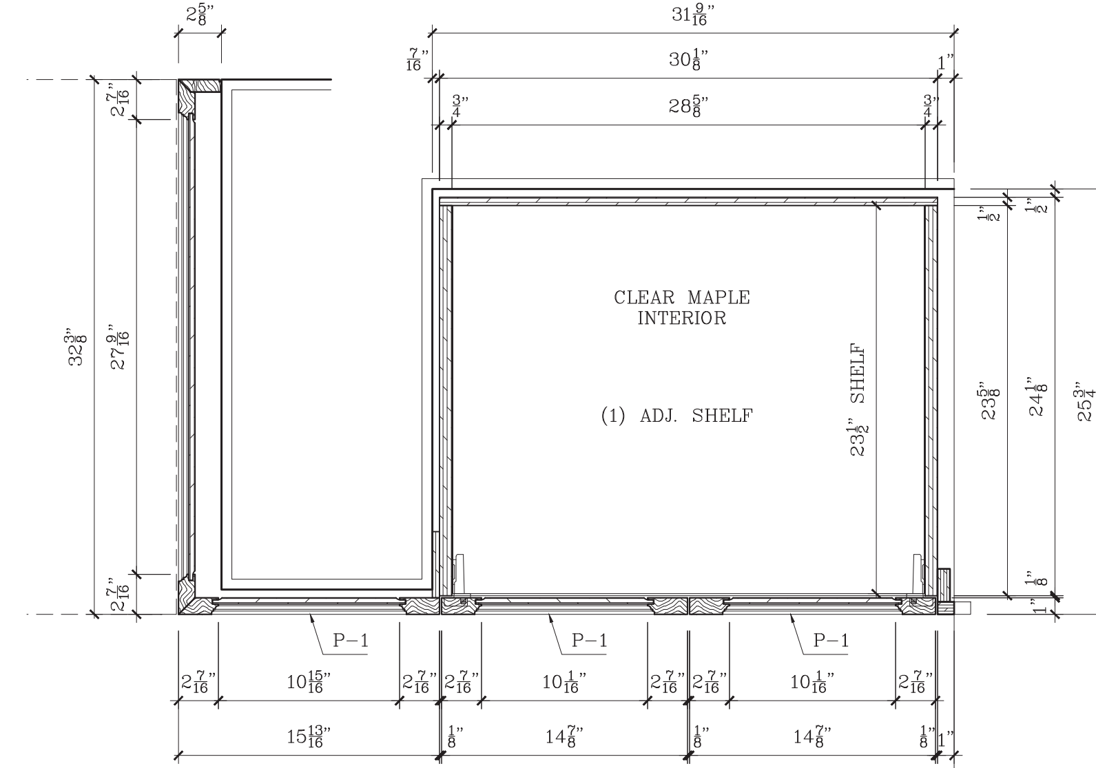
4 PLAN SECTION SCALE: 1-1/2"=1'-0"
