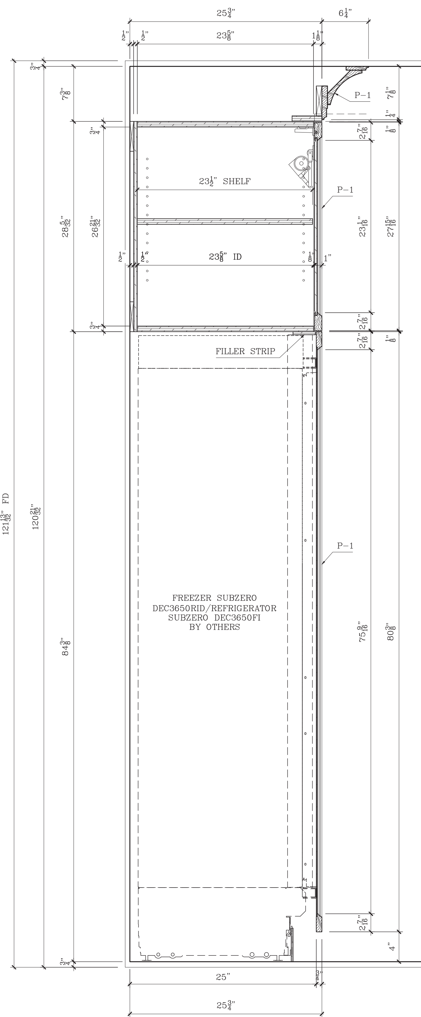
11 VERTICAL SECTION SCALE: 1-1/2"=1'-0"
