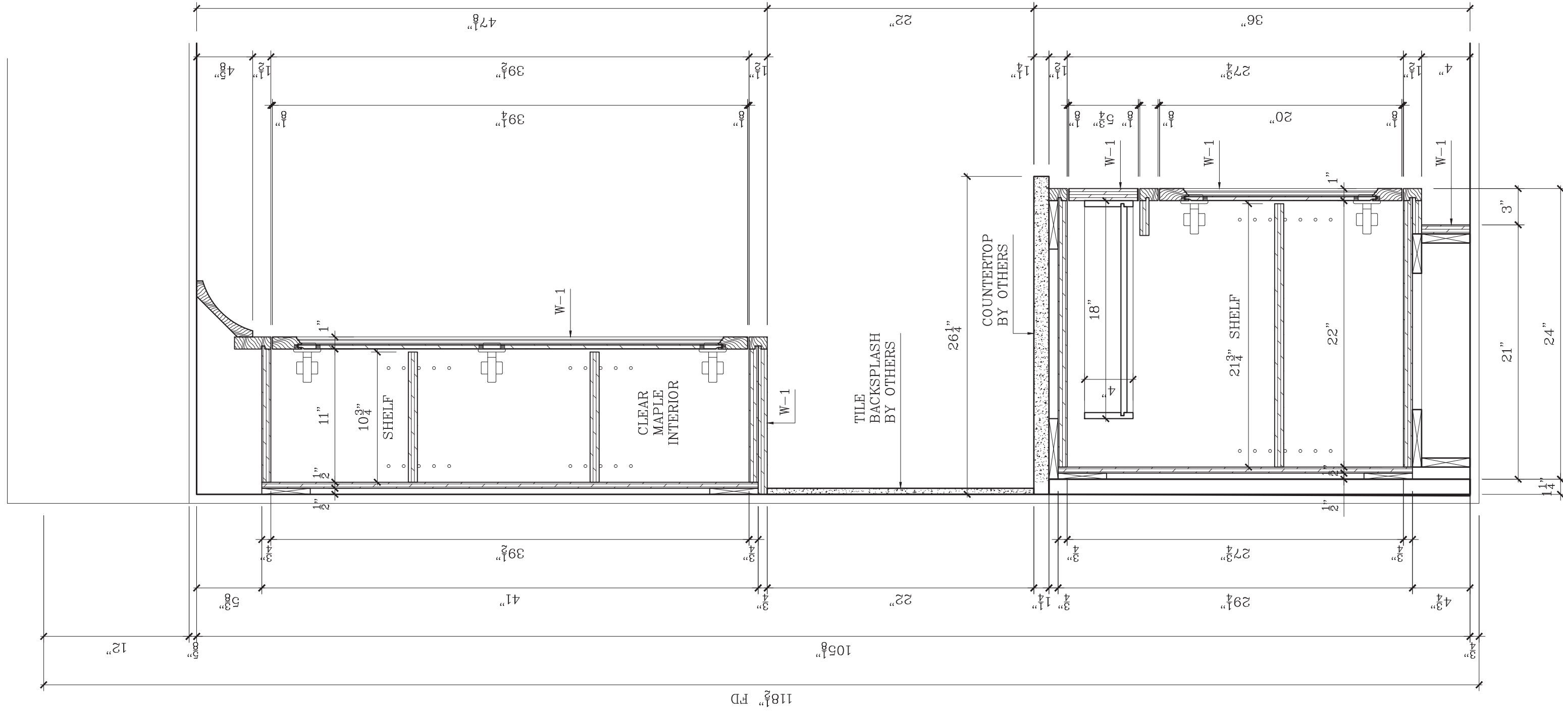
8 VERTICAL SECTION SCALE: 1-1/2"=1'-0"
