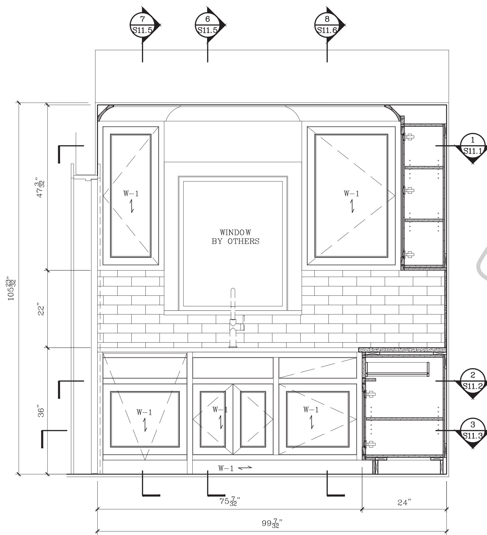
A ELEVATION SCALE: 3/4"=1'-0"
