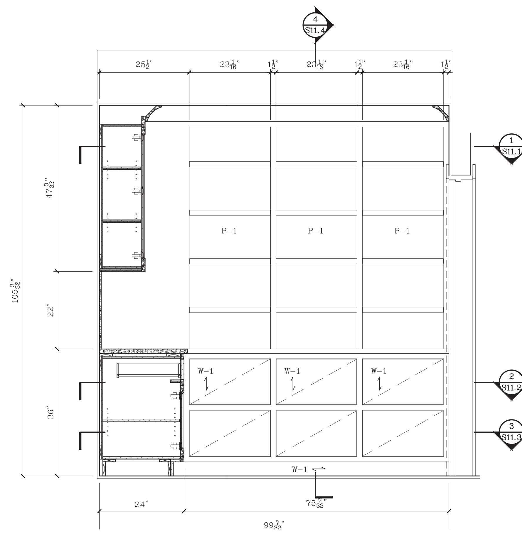
C ELEVATION SCALE: 3/4"=1'-0"
