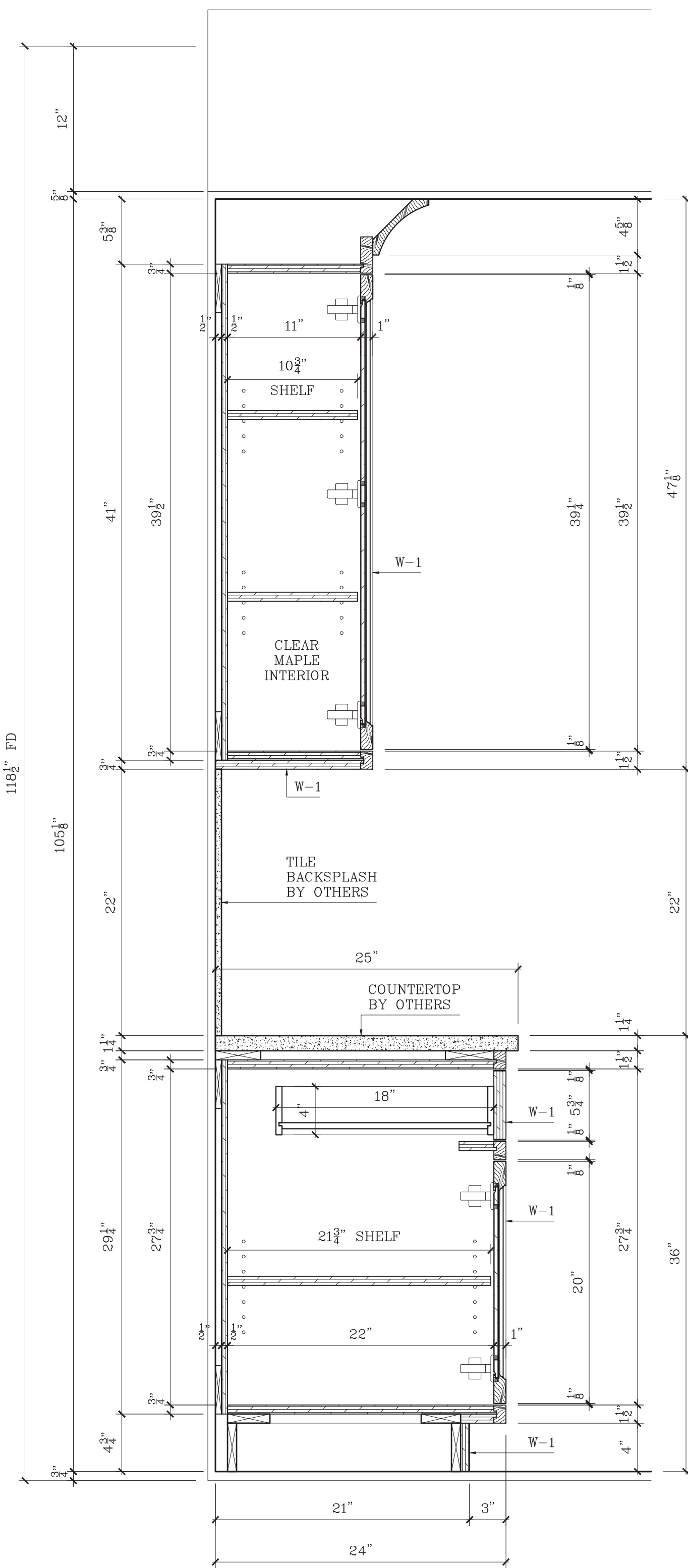
5 VERTICAL SECTION SCALE: 1-1/2"=1'-0"
